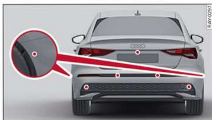
Fig. 95 Parte trasera: Sensores y cámaras
