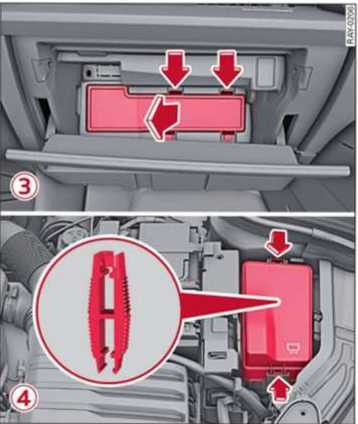
Fig. 186 Guanterera (vehículos con volante a la derecha): Cubierta ③. Lado izquierdo del compartimento del motor: Cubierta ④
