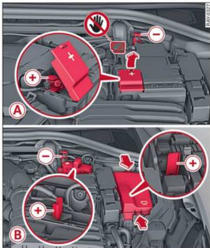
Fig. 181 Compartimento del motor: Conexiones para el cargador o cables de ayuda de arranque: A Vehículos con batería en el compartimento del motor, B Vehículos con borne de ayuda de arranque (+) en el compartimento del motor
