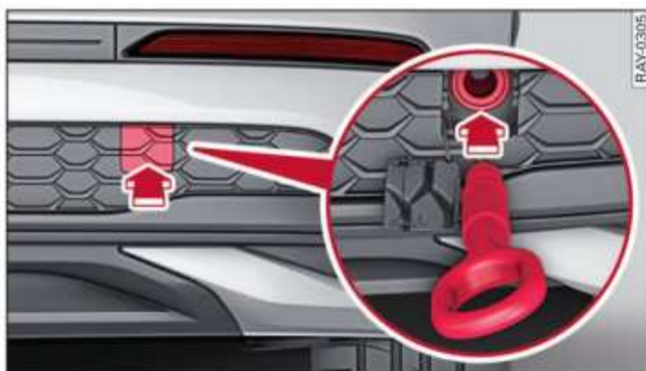
Fig. 184 Parachoques trasero: Enroscar la argolla de remolque
