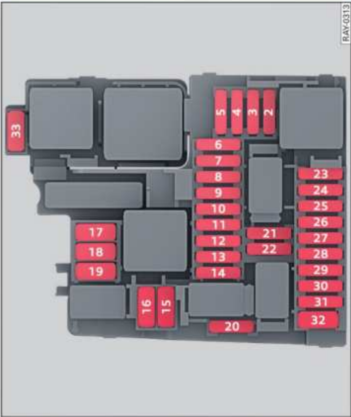
Fig. 188 Compartimento del motor, izquierda: Dotación de fusibles
