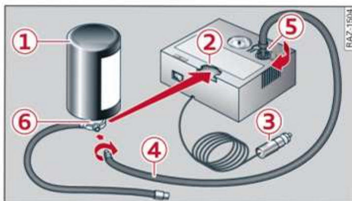
Fig. 172 Componentes del juego para reparación de neumáticos
