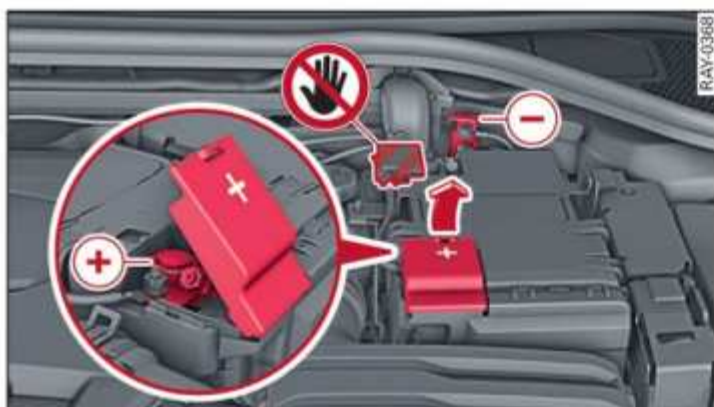
Fig. 162 Compartimento del motor: Conexiones para cargador o cable de ayuda de arranque
