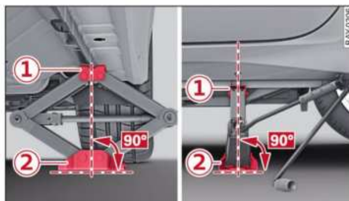
Fig. 178 Larguero inferior: Colocar el gato
