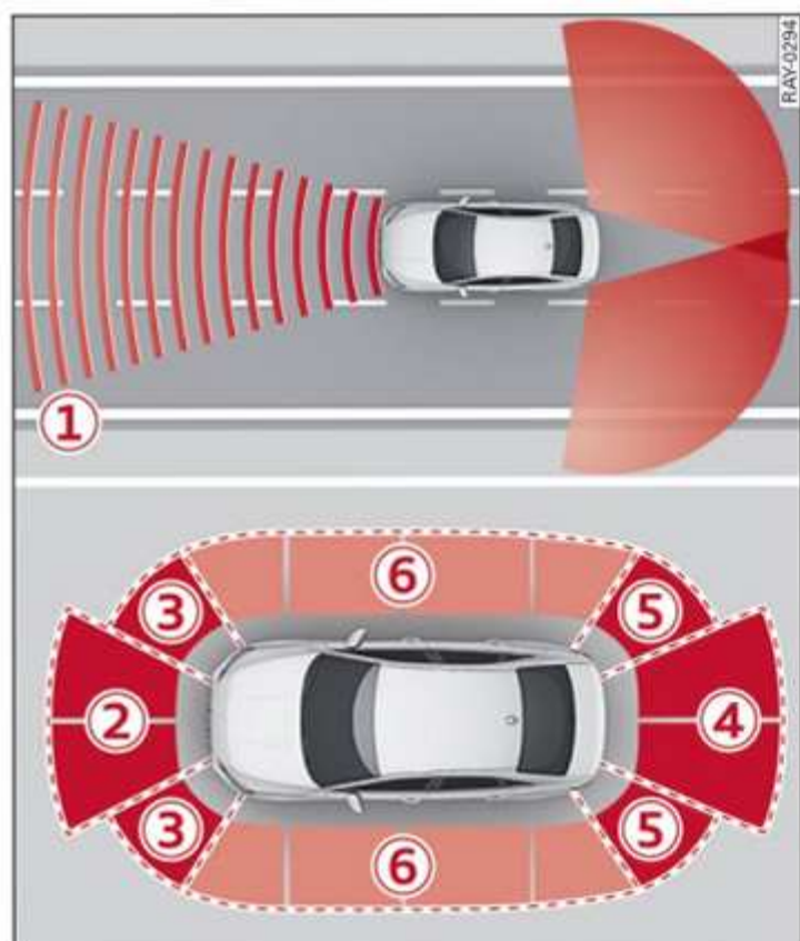
Fig. 92 Zonas de detección de los sensores
